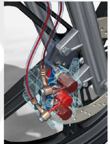
FREIO MECÂNICO E HIDRÁULICO
