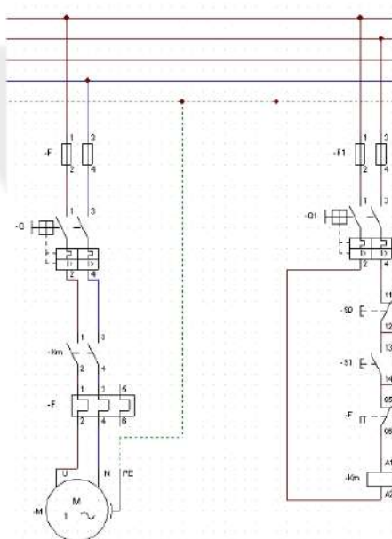
INTERPRETAÇÃO E LEITURA DE DIAGRAMAS DE COMANDOS
